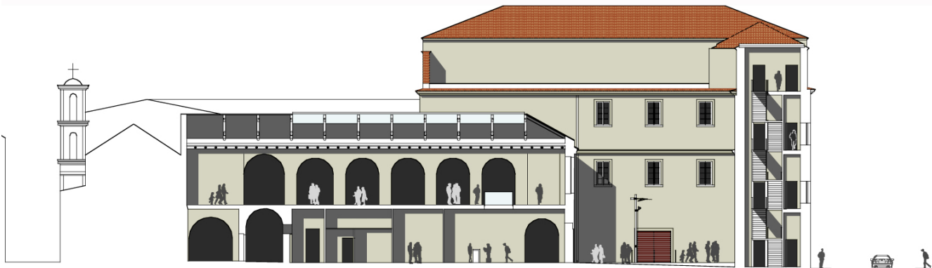
Sezione longitudinale
