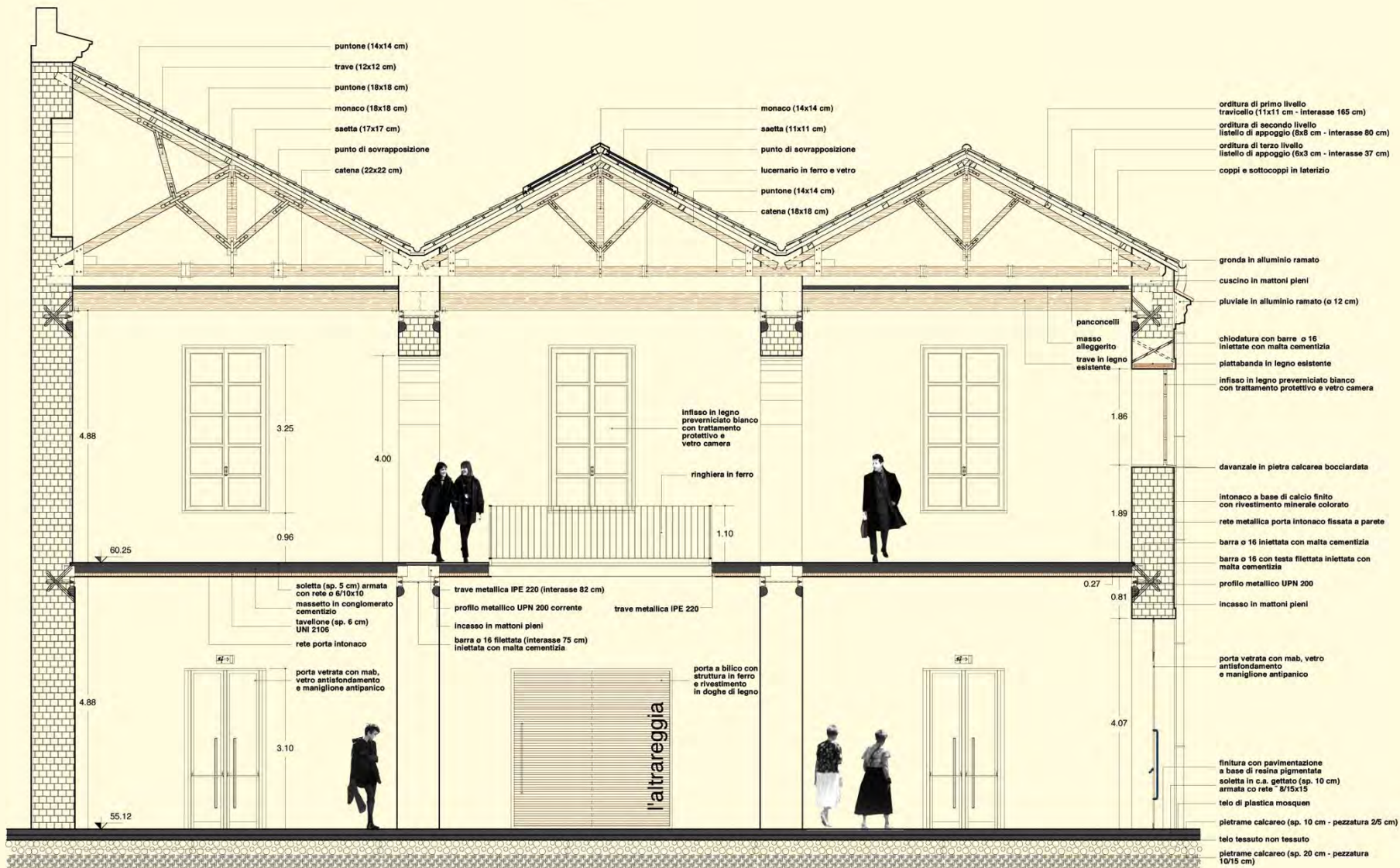
PARTICOLARE A
